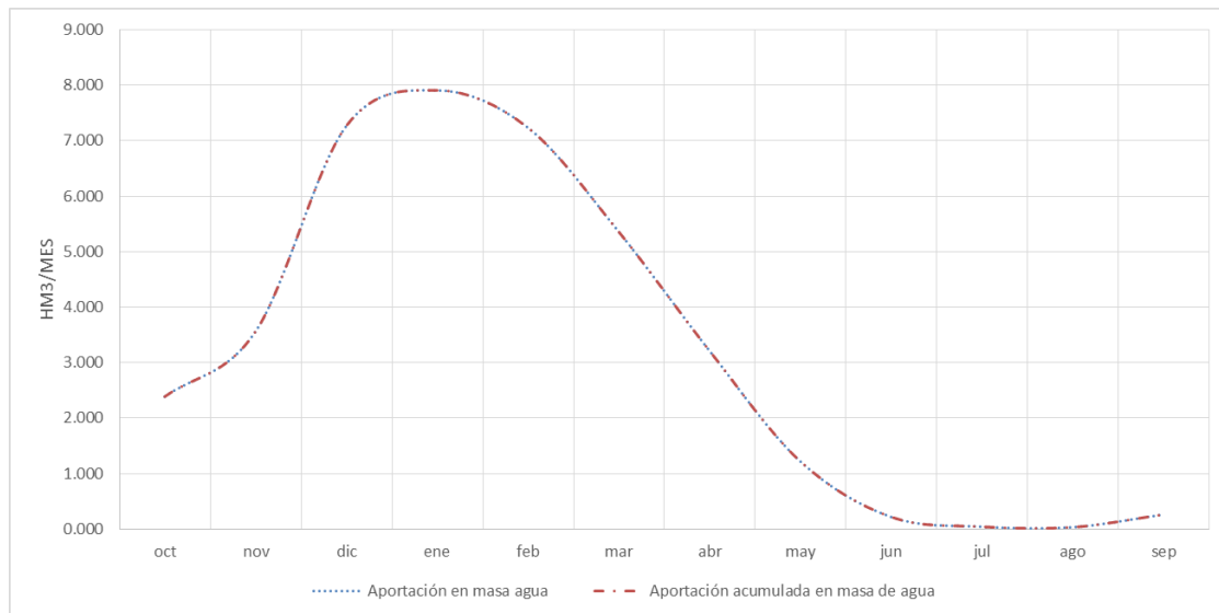
Aportación media y acumulada anual
